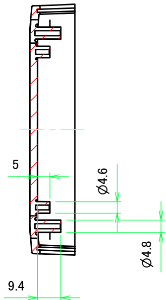
C-C ( 1 : 1.5 )
